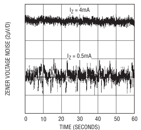
Zener Noise
