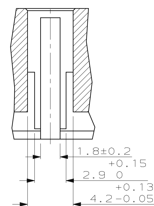
SECTION DD
