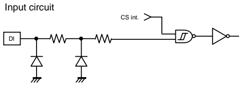
Fig.73 Input circuit (DI)
