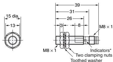
Diagram 28 E2E-X2D□-M3G/E2E-X1R5E□-M3/X1RF□-M3
