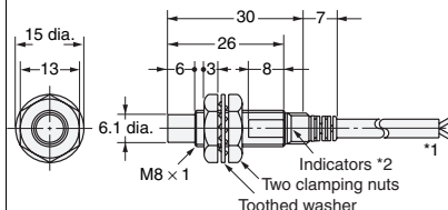
Diagram 6 E2E-X4MD E2E-X2ME /F
