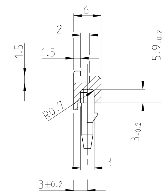
Schnitt C-C SECTION C-C
