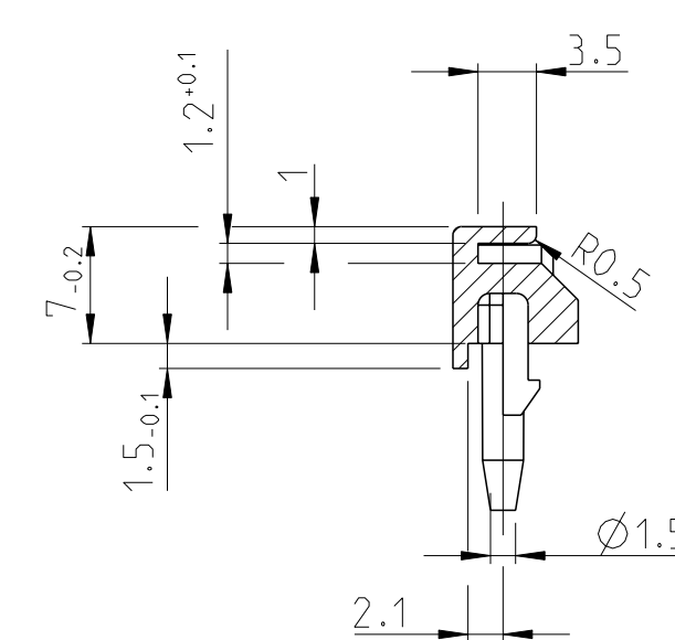
Schnitt B-B SECTION B-B
