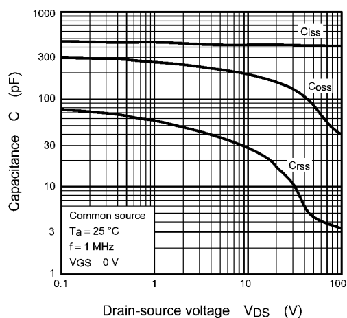
Fig. 8.3 C - V_{DS}
