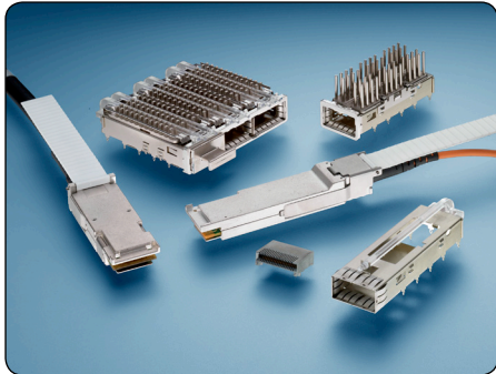
QSFP/ QSFP+ 产品
