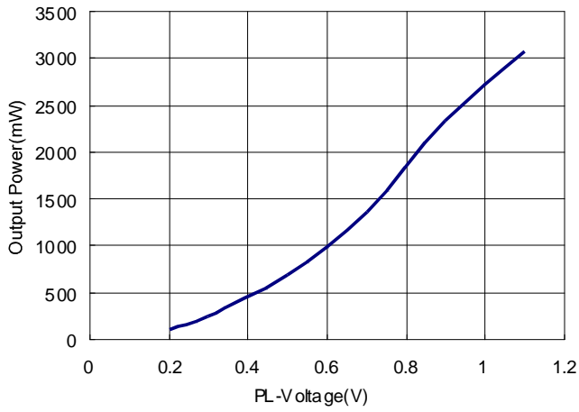
19. Output Power VS PL-Voltage
