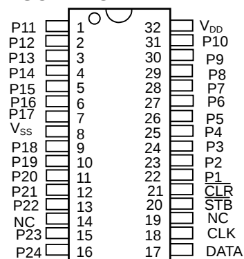
NJU3719AV
