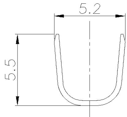
SEC. A-A
