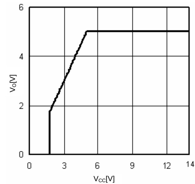
Fig.15 V_{CC}-V_O ( I_O=0\text{mA} )
