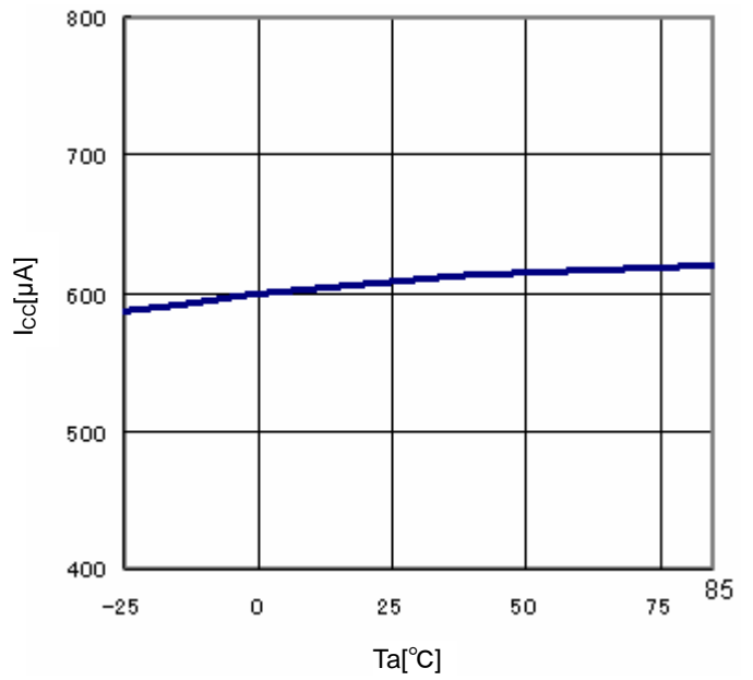
Fig.10 T_a - I_{cc}
