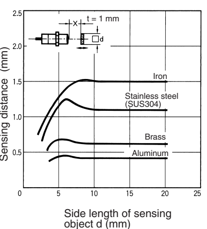
E2E-X1R5E/V E2E-X1R5Y
