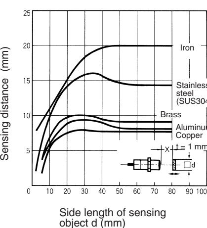
E2E-X20MD
