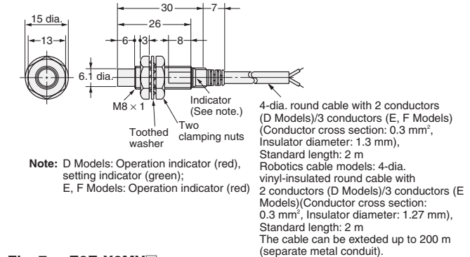
Fig. 7 : E2E-X2MY□
