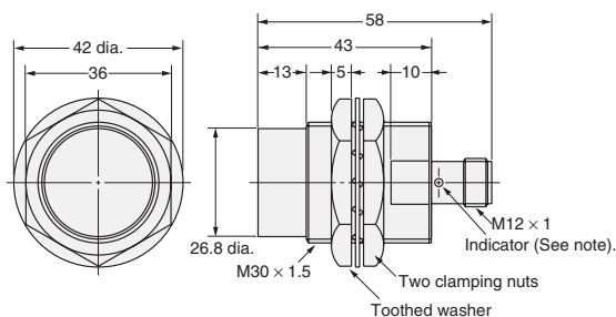
Fig. 26 : E2E-X20MD□-M1(G)/E2E-X18ME□-M1/F□-M1 E2E-X18MY□-M1
