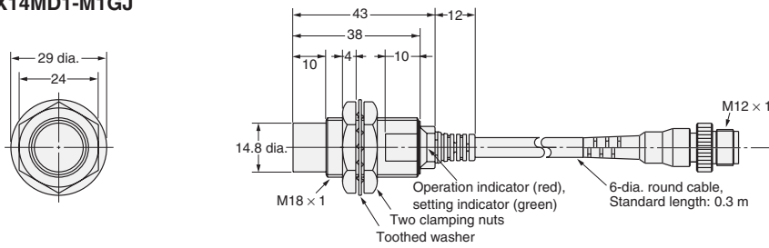
Fig. 33 : E2E-X14MD1-M1GJ
