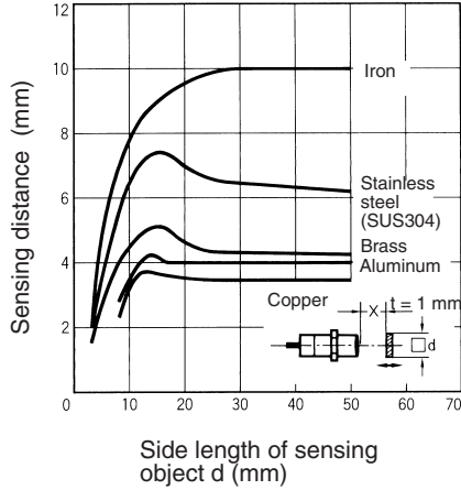
E2E-X14MD
