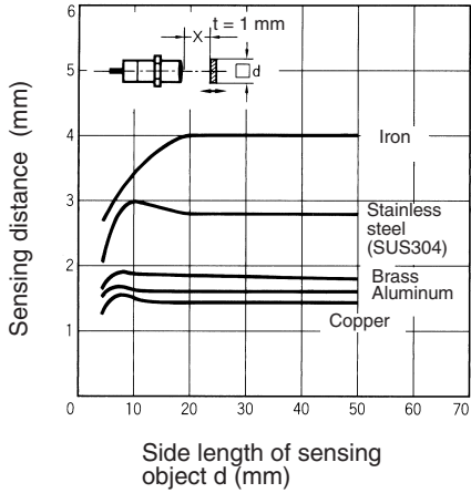
E2E-X20MD
