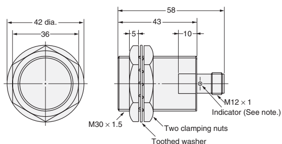
Fig. 25 : E2E-X10D□-M1(G)/E2E-X10E□-M1/F□-M1 E2E-X10Y□-M1
