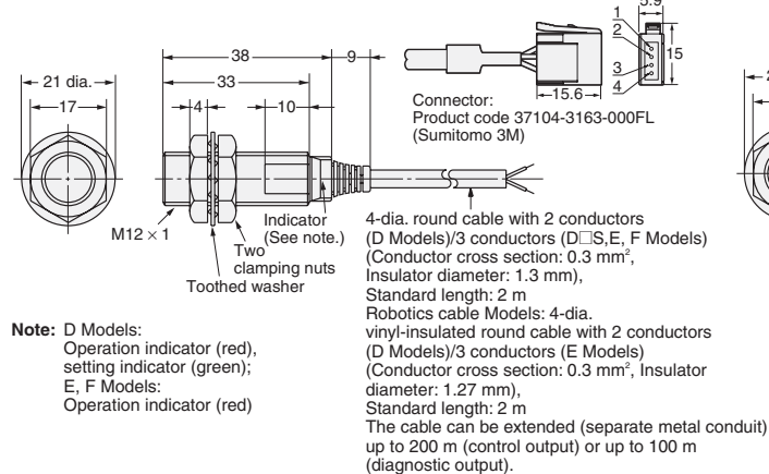
Fig. 8 : E2E-X3D□-N E2E-X2E□/F□
