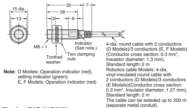
Fig. 6 : E2E-X1R5Y□
