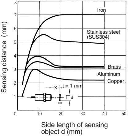
E2E-X8MD
