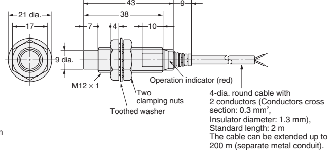
Fig. 11 : E2E-X5MY□
