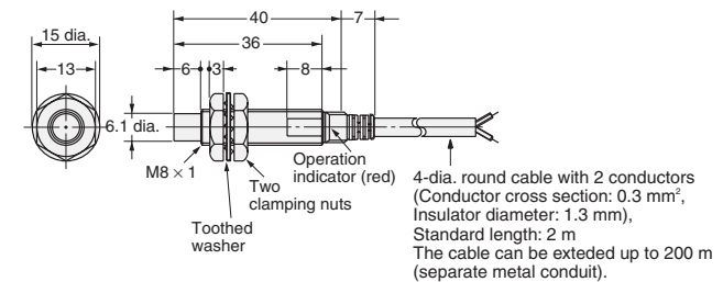
Fig. 9 : E2E-X8MD□ E2E-X5ME□/F□
