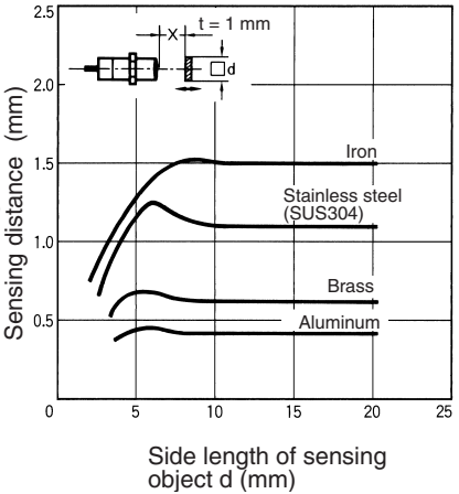
E2E-X1R5E/V E2E-X1R5Y
