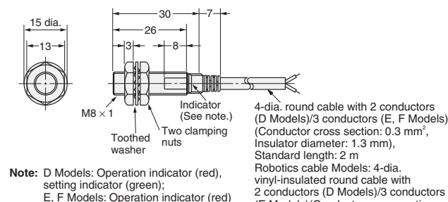
Fig. 4 : E2E-X2D□-N E2E-X1R5E□/F□
