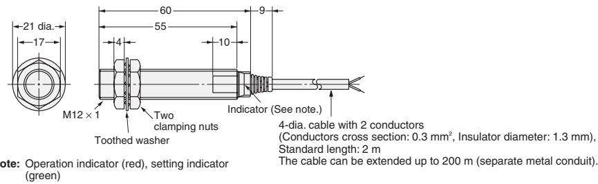
Fig. 13 : E2E-X7D□-N/ E2E-X5E□/F□ E2E-X5Y□/E2E-X7T1
