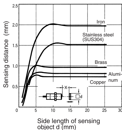
E2E-X2ME□/F□ E2E-X2MY□
