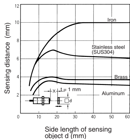
E2E-X10ME□/F□ E2E-X10MY□
