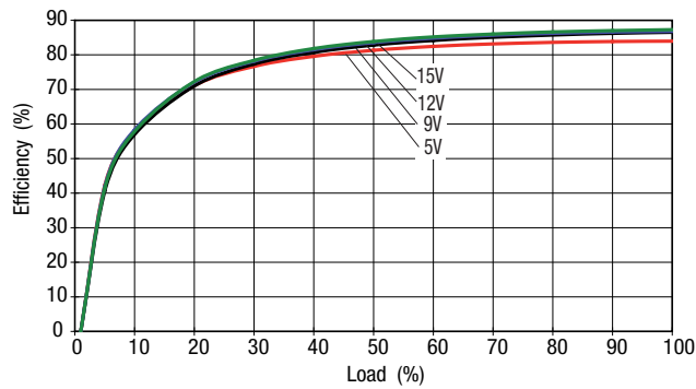
MEV1x05xxDC
