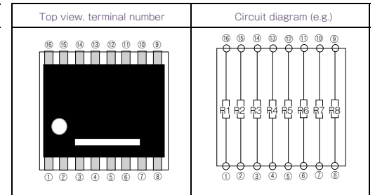
RM10280(10.2mm×7.2mm)
