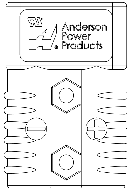
SB®175 - 2 Pole
