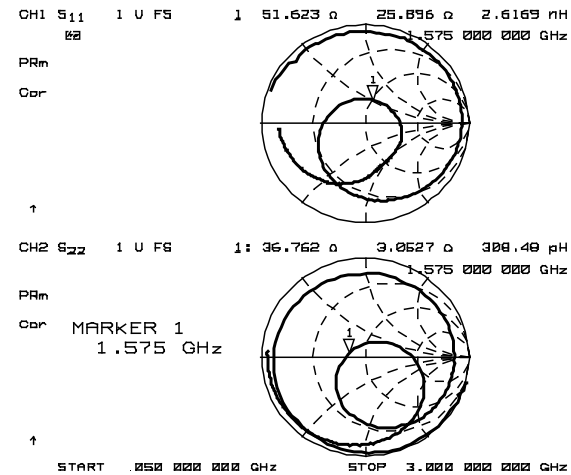
Zin, Zout
