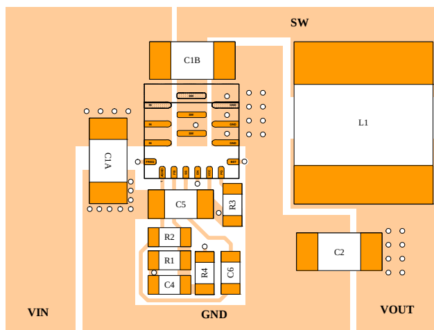
Top Layer
