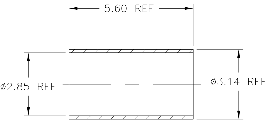
FERRULE
