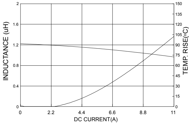
PA4345.122NLT
