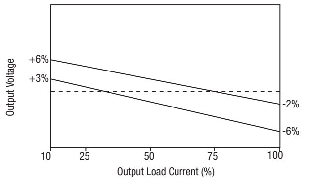
NXE2S1215MC
