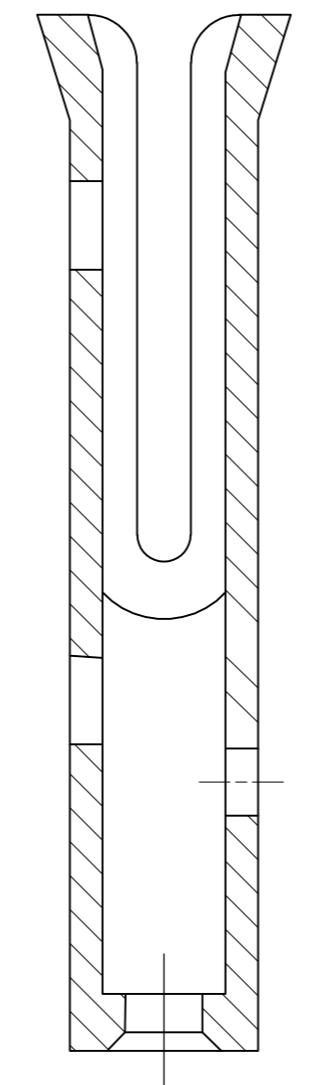
SECTION D-D
