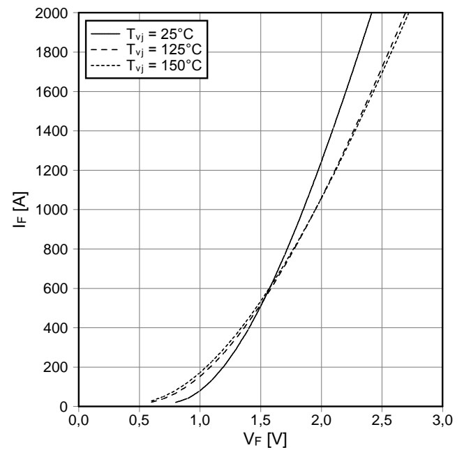
Durchlasskennlinie der Diode-Wechsler. (typisch) forward characteristic of diode-inverter (typical) I_F = f(V_F)
