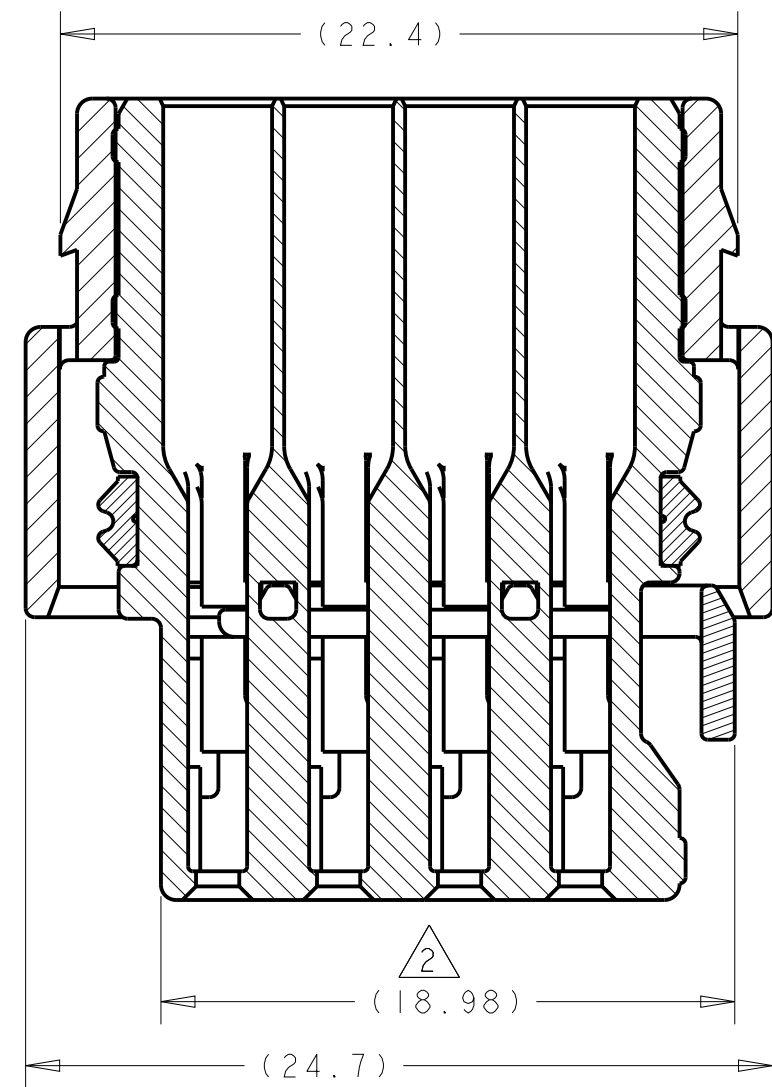
SECTION A-A
