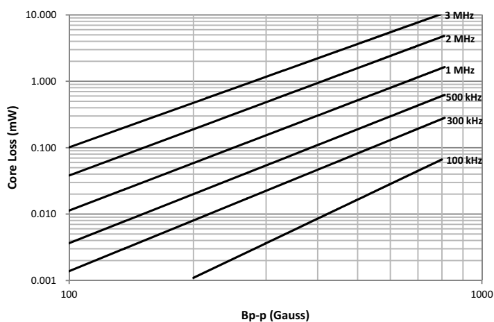
MPI2512V2-R68-R
