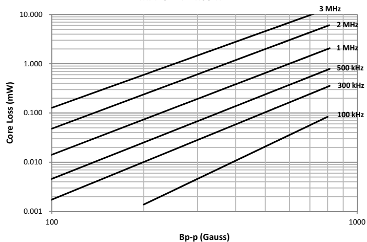
MPI2512V2-R68-R
