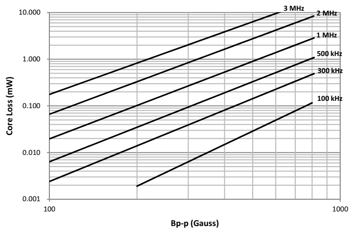
MPI2512V2-1R0-R
