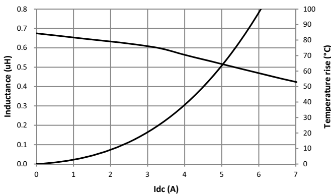
MPI2512V2-R68-R
