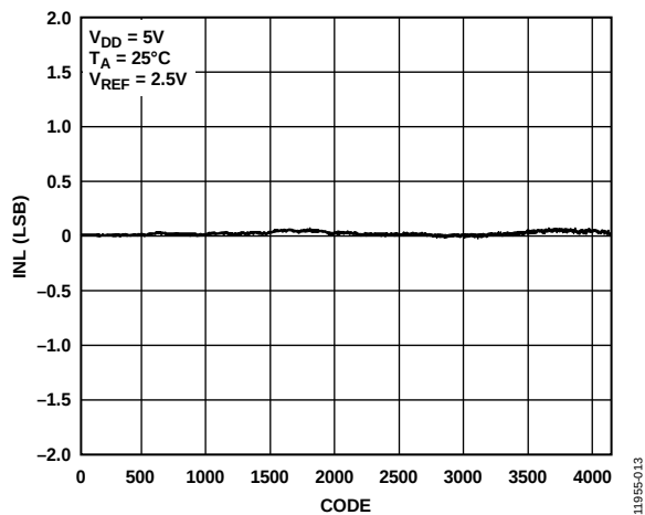
Figure 13. AD5681R INL
