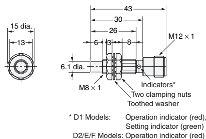
Diagram 19 E2E-X4MD□-M1(G) E2E-X2ME□-M1/E2E-X2MF□-M1
