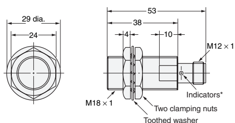
Diagram 24 E2E-X7D□-M1(G)/E2E-X5E□-M1/X5F□-M1 E2E-X5Y□-M1
