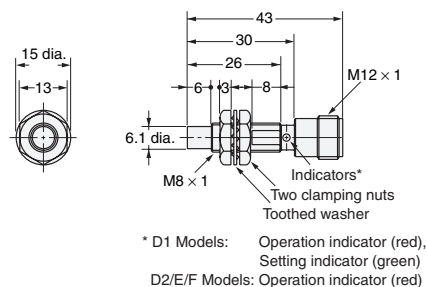
Diagram 19 E2E-X4MD□-M1(G) E2E-X2ME□-M1/E2E-X2MF□-M1
