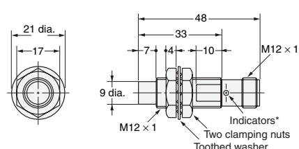
Diagram 21 E2E-X8MD□-M1(G) E2E-X5ME□-M1/E2E-X5MF□-M1
