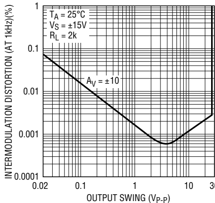
LT1169 • TPC26
