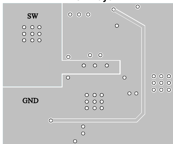
Inner2 Layer
