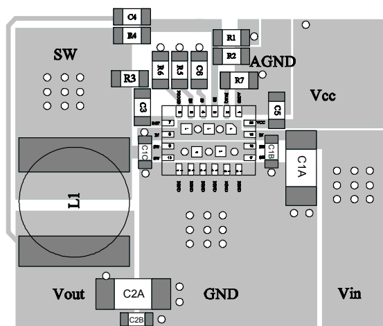
Top Layer
