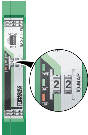
Bild 4 Thumb wheel
