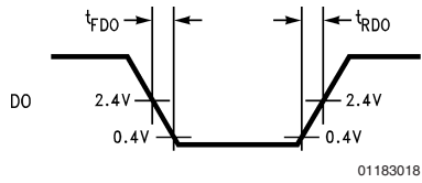
DO Falling and Rising Edge
