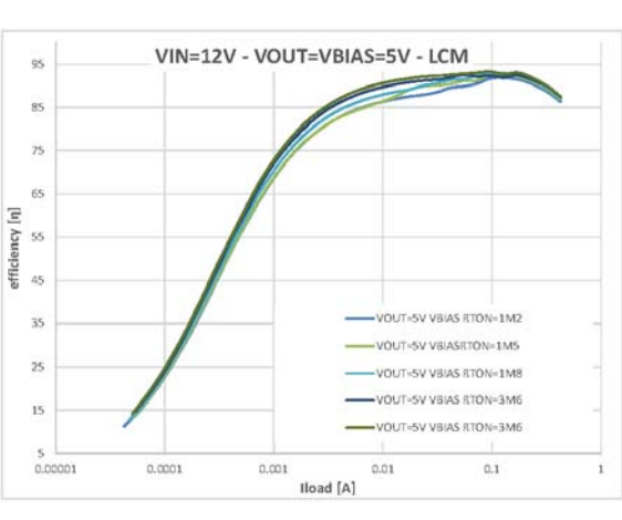
Figure 34. VIN 12 V - VOUT 5 V (log scale)
