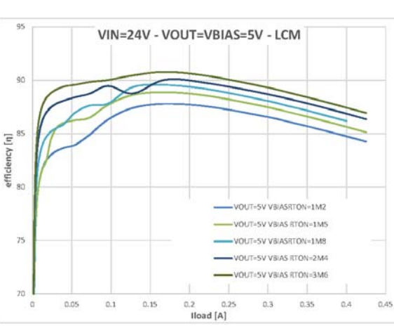
Figure 32. VIN 24 V - VOUT 5 V (linear scale)
