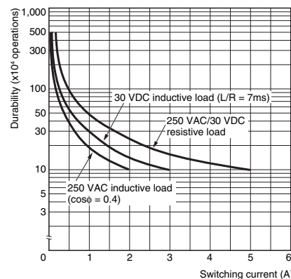
G2R-1Z, G2R-1AZ
