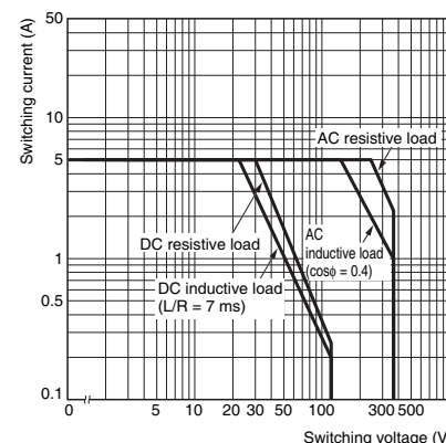
G2R-1Z4, G2R-1AZ4
