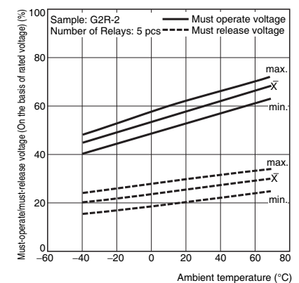
G2R-2
