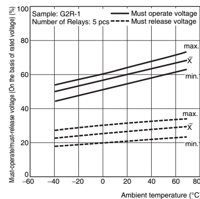
G2R-1
