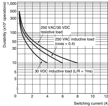
G2R-14, G2R-1A4
