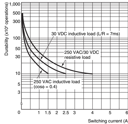
G2R-24, G2R-2A4
