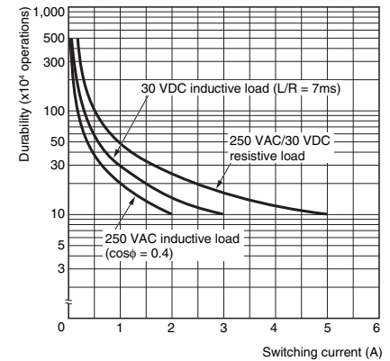
G2R-1Z4, G2R-1AZ4
