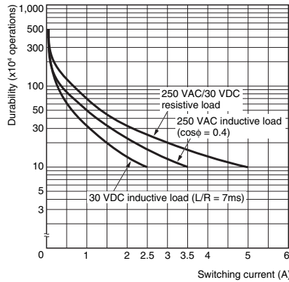
G2RK-1A, G2RK-1
