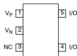
SOT-553
