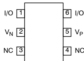
TSOP-6
