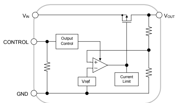
NJU7741
