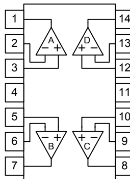
NJM074C / NJM084C NJM074CA / NJM084CA
