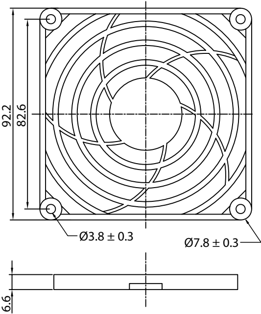
FAN GUARD
