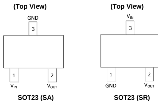
SOT23 (SA)
