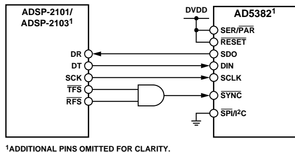
Figure 37. AD5382-to-ADSP-2101/ADSP-2103 Interface
