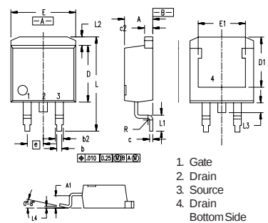
TO-263 AA Outline
