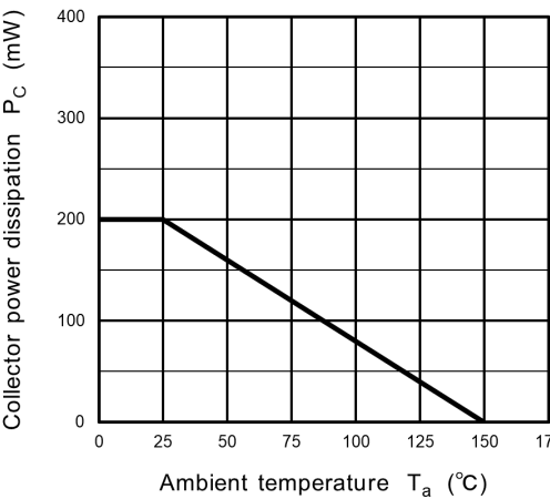
Fig. 6.4 P_C - T_a
