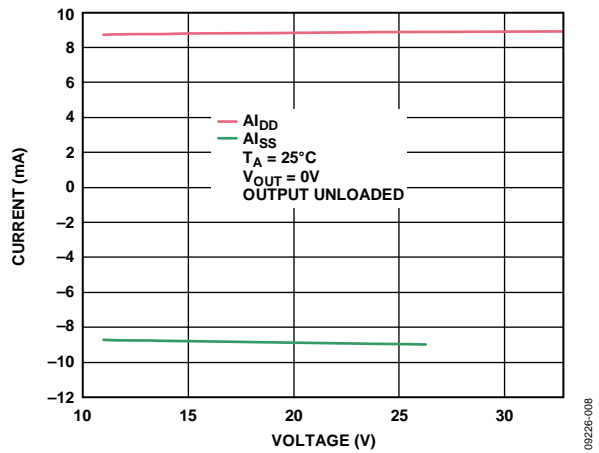
Figure 67. AI DD /AI SS vs. AV DD /AV SS
