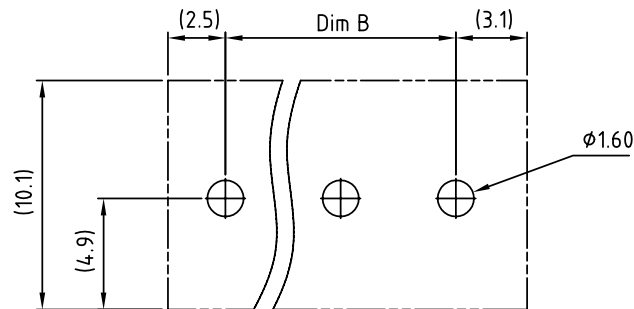
P.C.B LAYOUT
